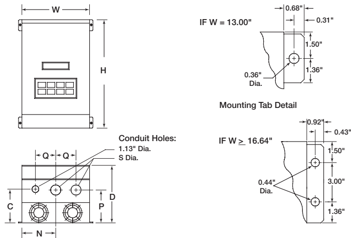
CONDUIT HOLES FOR 174578.00
